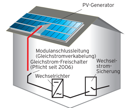
Abb. 23: PV-Anlage (schematisch)
